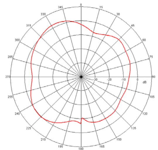
YZ-plane @2450MHz Total
