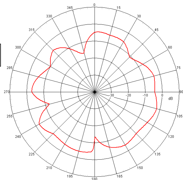
XZ-plane @868MHz — Total
