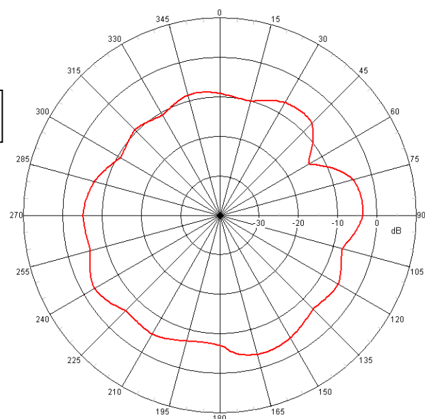
YZ-plane @868MHz — Total
