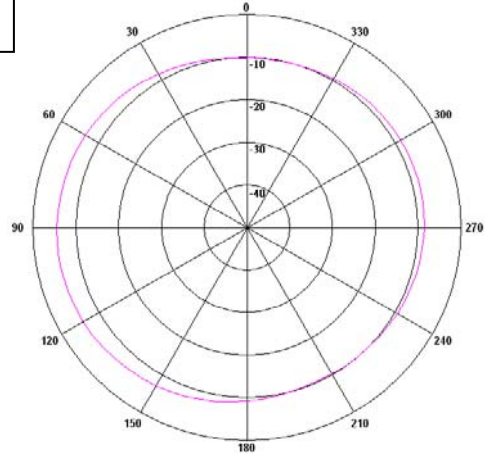
XZ cut @490MHz — Total
