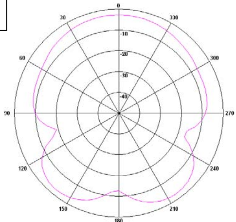
YZ cut @490MHz — Total
