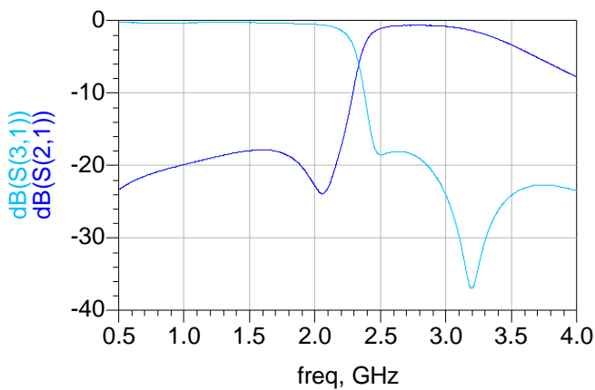
Attenuation
