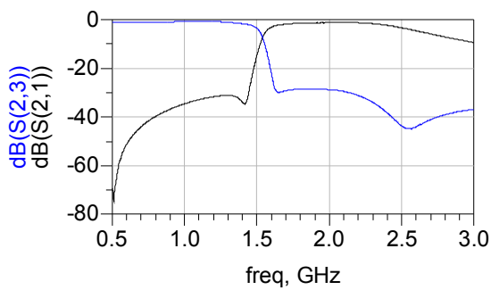
Attenuation
